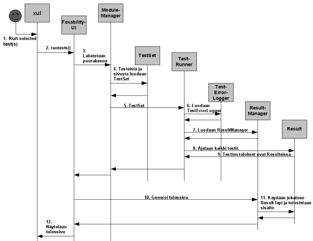
Kuva 4.3: Sekvenssikaavio testin ajamisesta.
