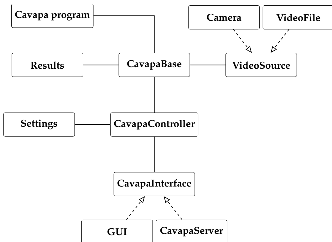
Kuva 3.1: CAVAPA-GUI-sovelluksen kokonaisrakenne.
