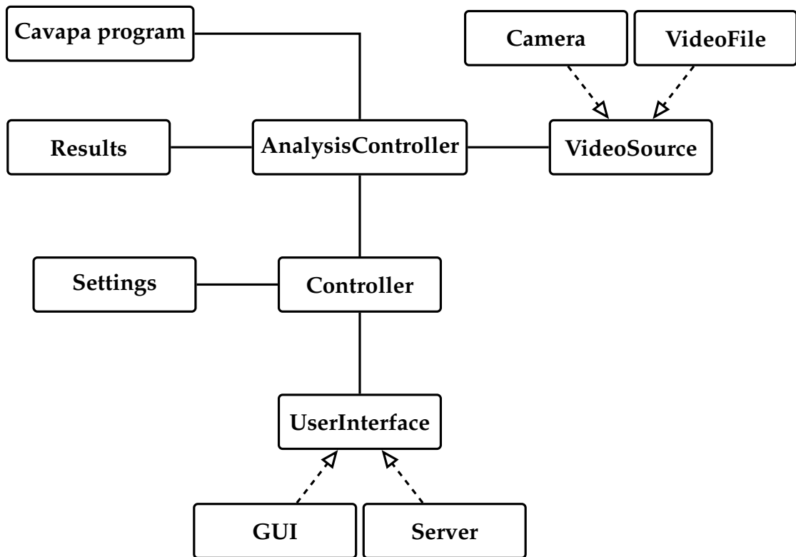
Kuva 3.1: CAVAPA-GUI-sovelluksen kokonaisrakenne.
