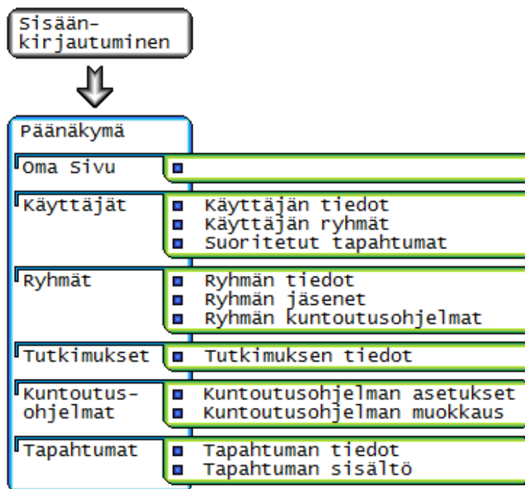
Kuva 3.1: Tutkijan käyttöliittymän näkymäkarta.
