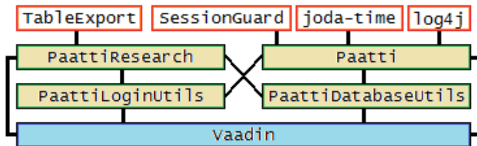
Kuva 5.2: Tietojärjestelmän rakenne.
