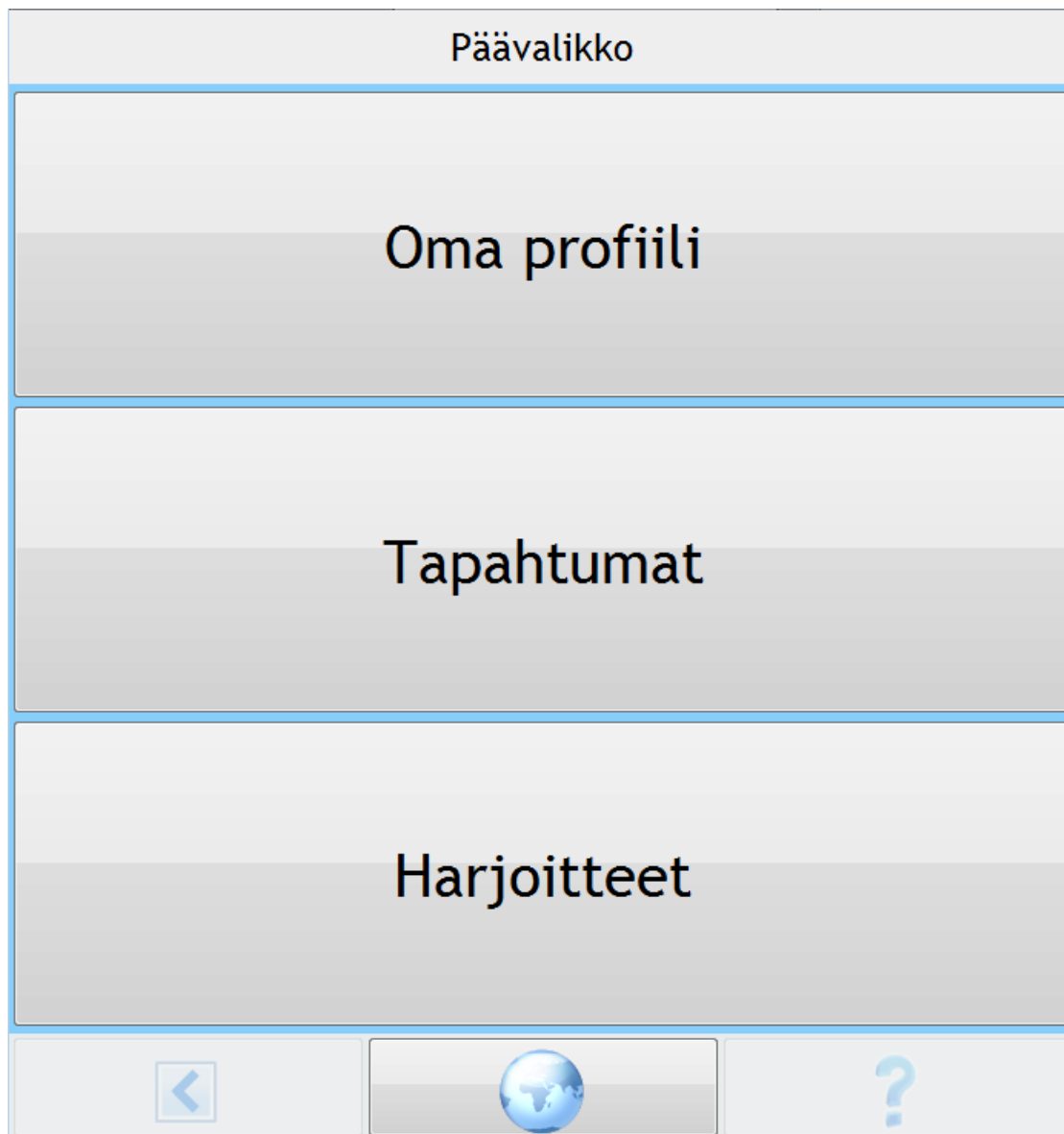
Kuva 4.5: Sovelluksen päävalikko.
