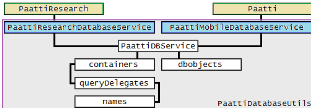
Kuva 5.5: PaattiDatabaseUtilsin rakenne.
