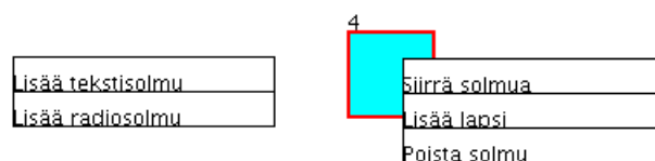
Kuva 3.15: Tapahtumamuokkaimen hiirivalikot.
