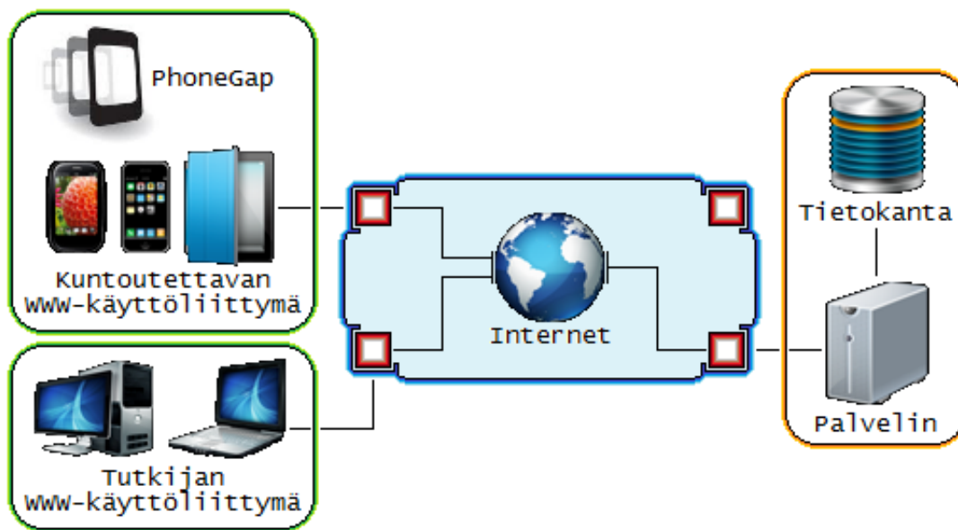
Kuva 5.1: Tietojärjestelmän asiakas-palvelinarkkitehtuuri.
