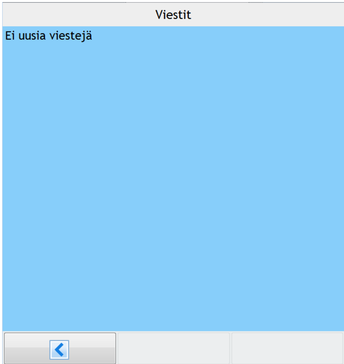
Kuva 4.16: Viestit -näky.
