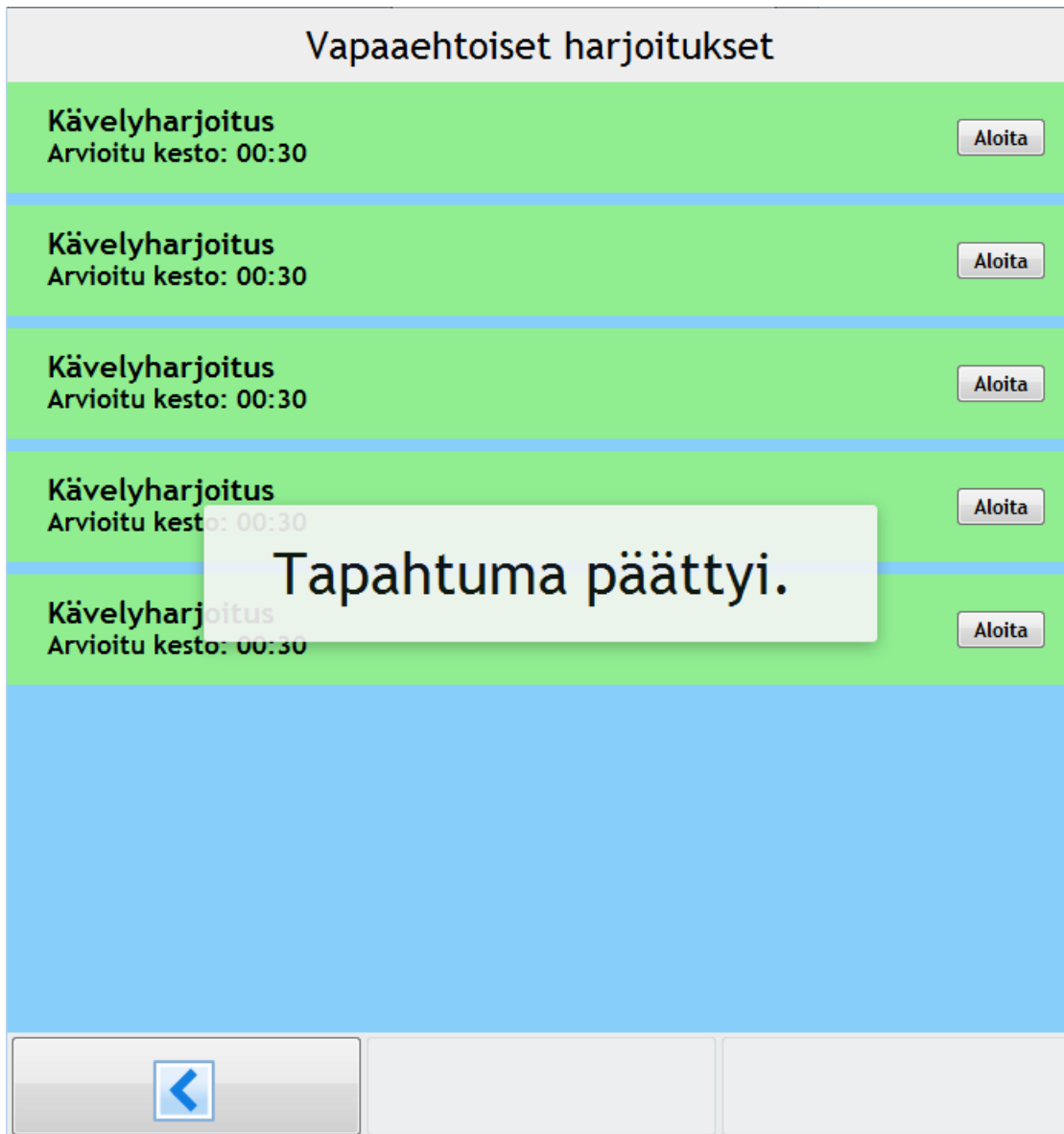
Kuva 4.13: Tapahtuman päätyminen.
