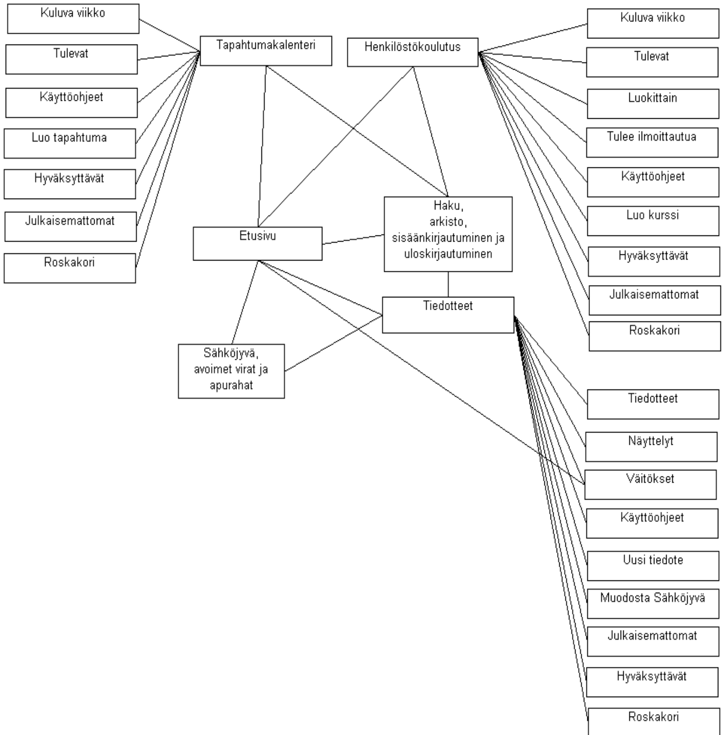
Kuva 6. Tiedottajan sivustokartta.
