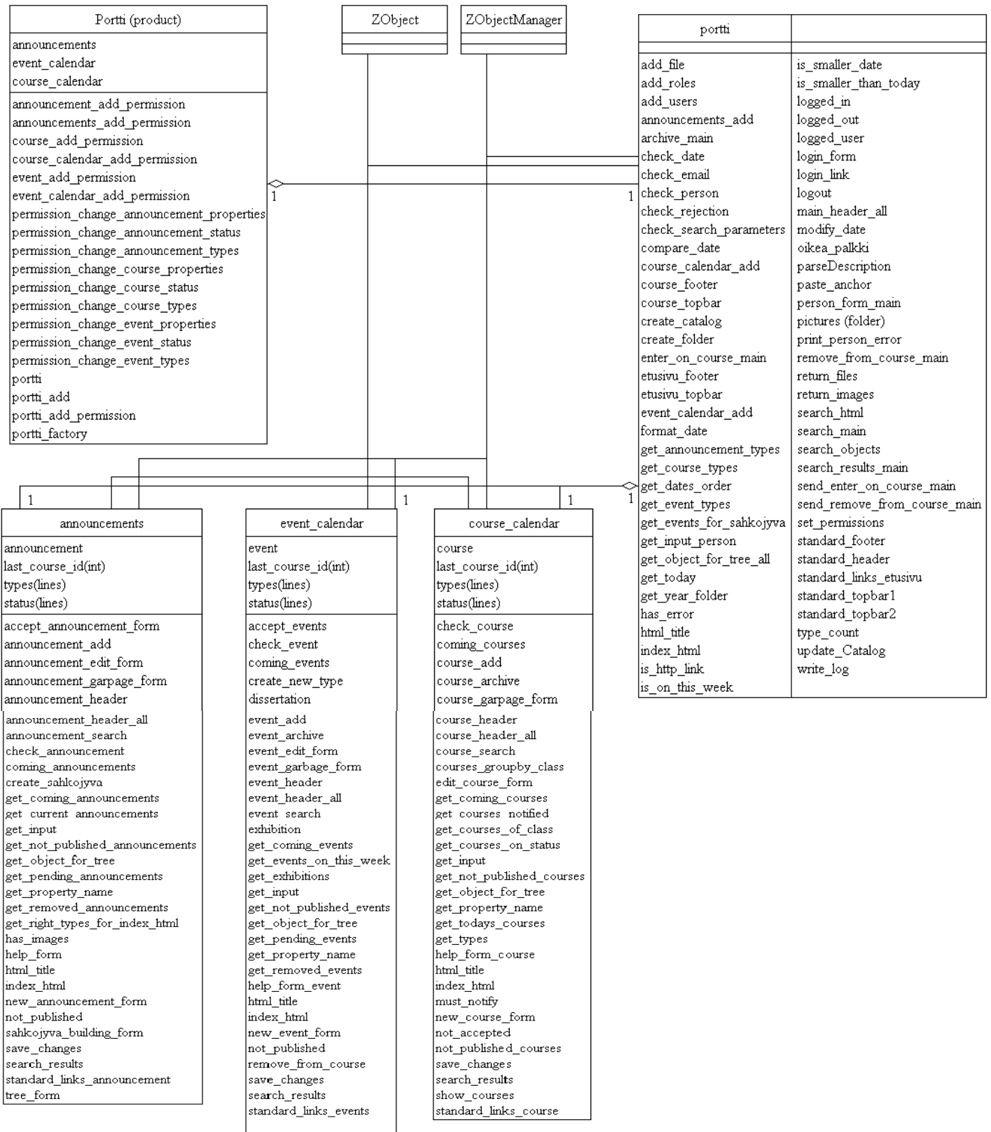
Kuva 2. Sovelluksen luokkarakenne.
