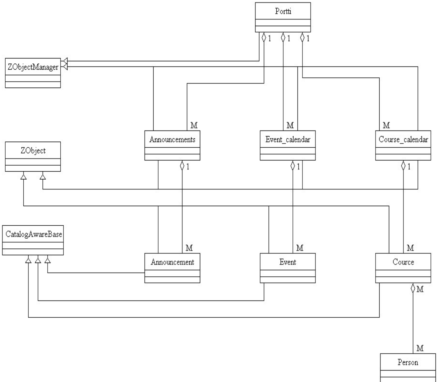
Kuva 2. Sovelluksen luokkarakenne.
