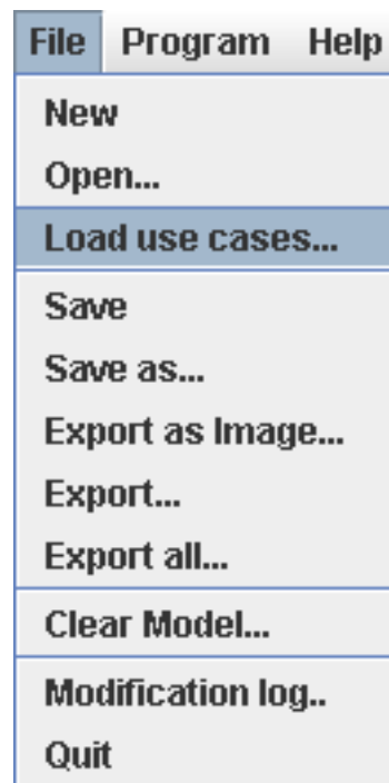
Kuva 1.1: Käyttötiedostojen lataaminen
