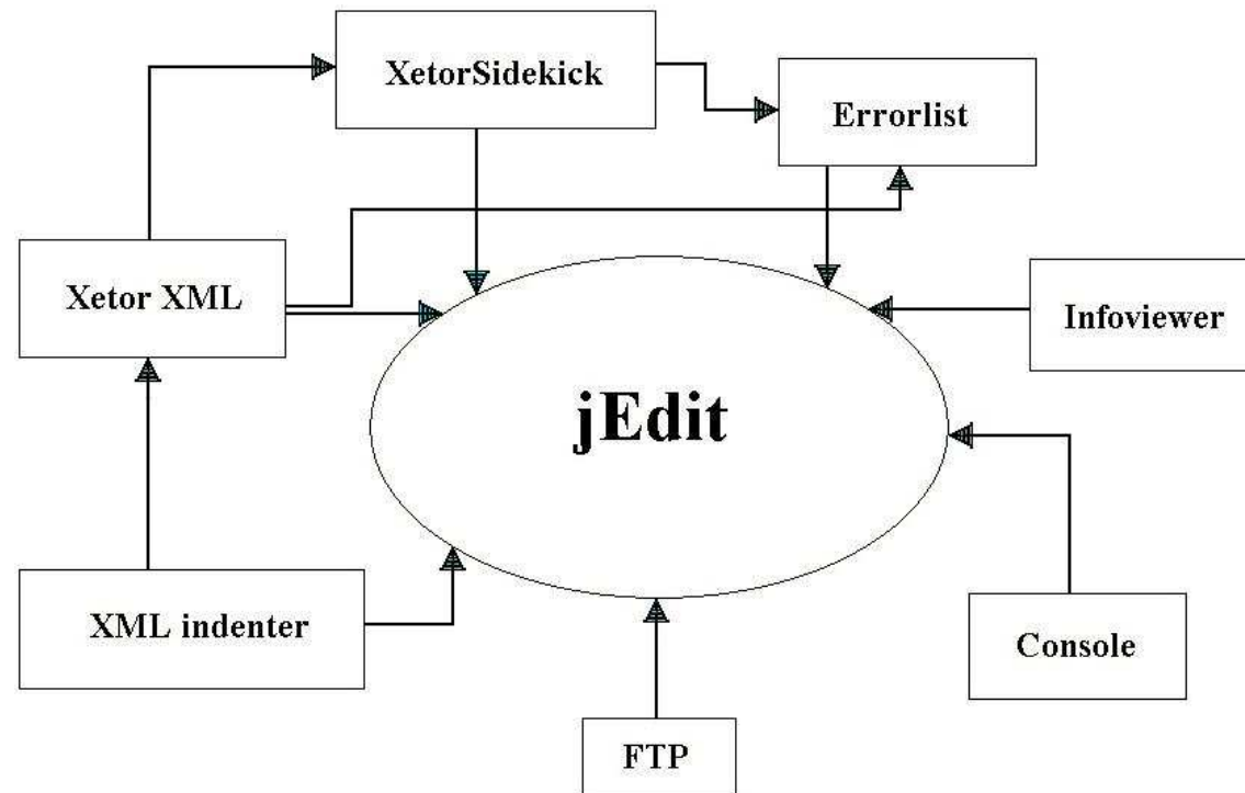
Kuva 1: Sovelluksen rakenne.
