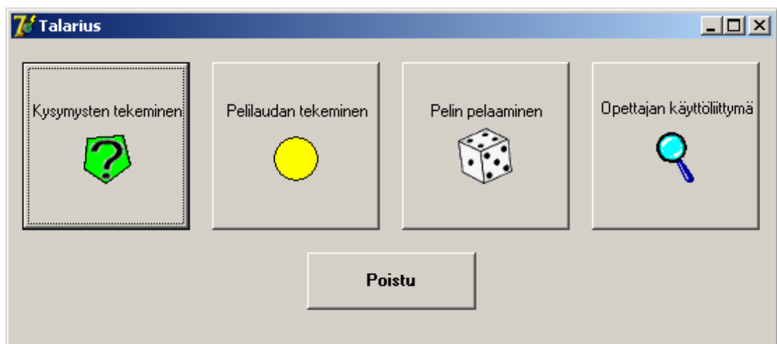
Kuva 4.1: Talarius -käyttöliittymä.
