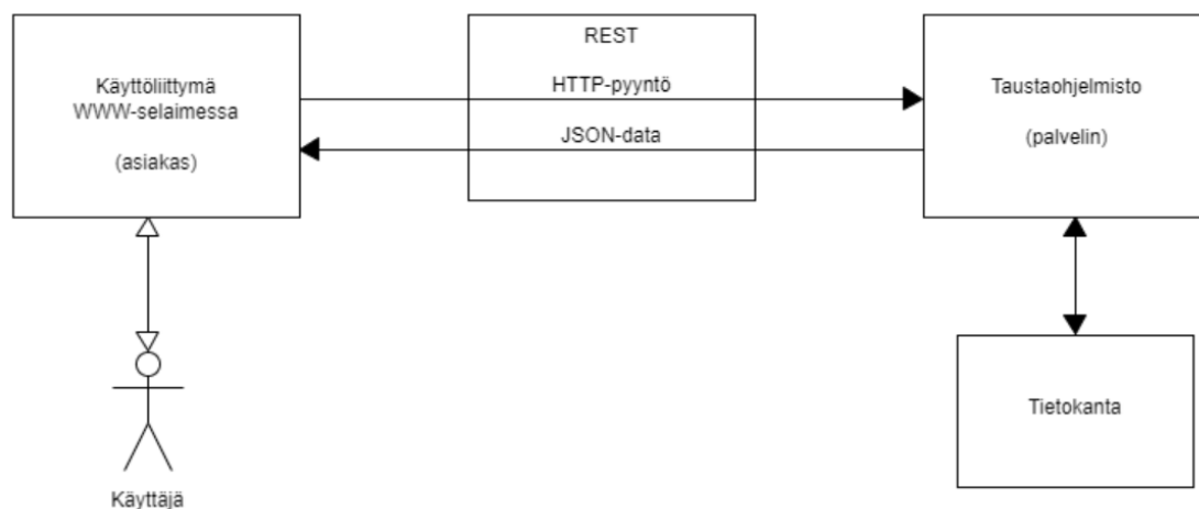
Kuva 4.1. Sovelluksen kokonaisrakenne.
