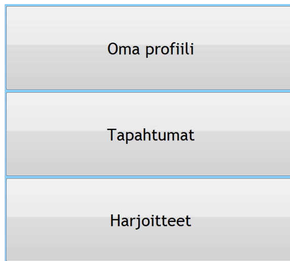
Kuva 4.3: Käyttöliittymän sisältöalue.
