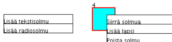
Kuva 3.15: Tapahtumamuokkaimen hiirivalikot.
