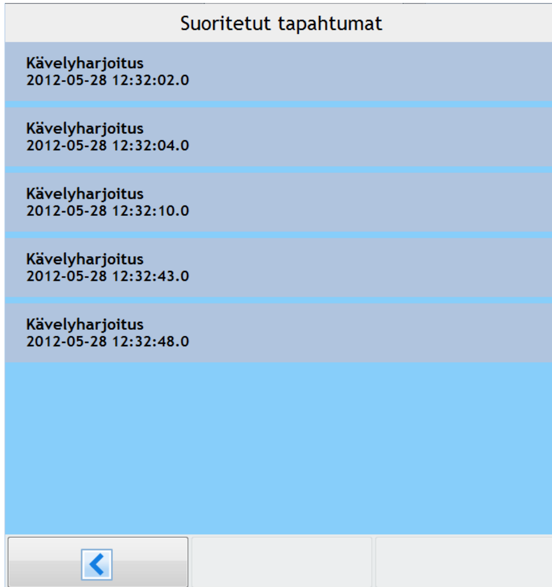
Kuva 4.7: Edistymisen -alavalikko.
